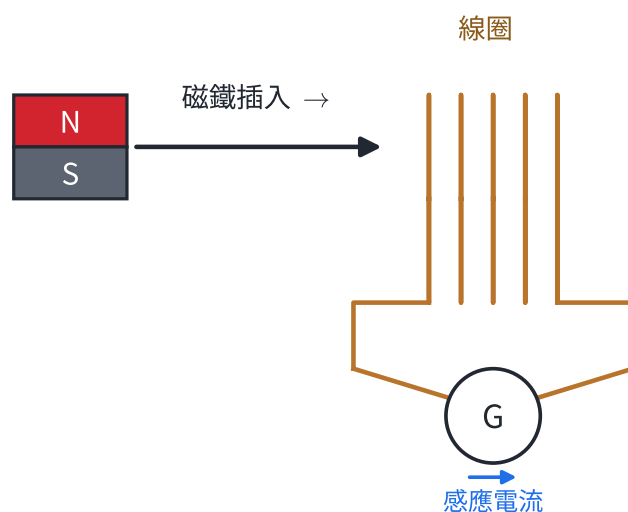
圖 4-3：電磁感應。磁鐵相對線圈運動（如插入）時，穿過線圈的磁場發生變動，線圈中產生感應電流（電流計 G 偏轉）。磁鐵靜止時則無感應電流。
